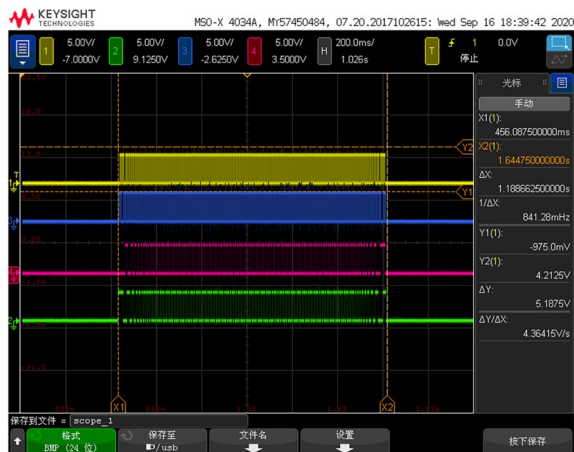
图 12 调焦电机调整时间
