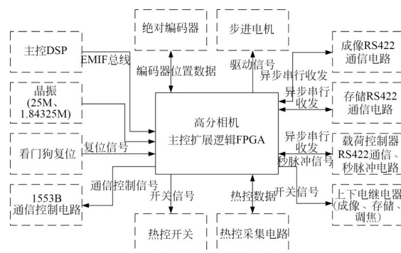
图1 主控接口扩展逻辑FPGA外部接口
