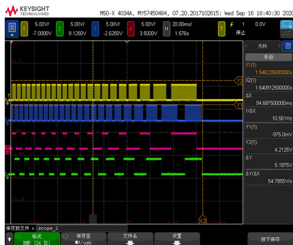
图 13 调焦电机减速段
