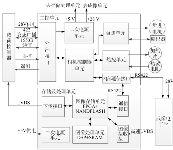
图 3 系统总体功能框图
