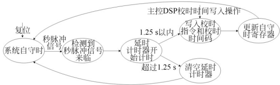
图 8 时间码校时守时示意图 Fig.8 Schematic diagram of time code correction and punctuality
