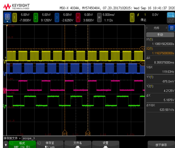
图 14 调焦电机匀速段
