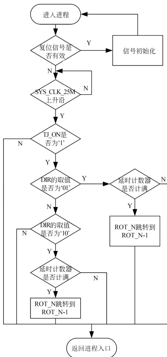
图 6 调焦电机模块内部单元结构
