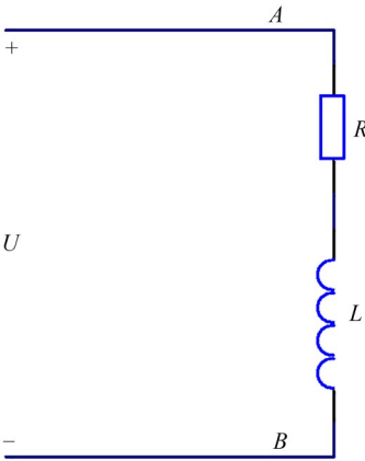
图 4 步进电机 AB 相电路
