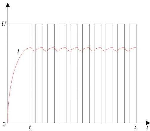
图 5 驱动波形及电流示意图
