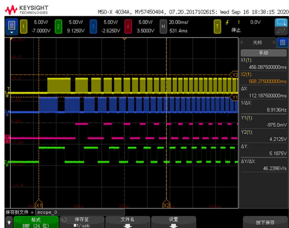
图 11 调焦电机加速段
