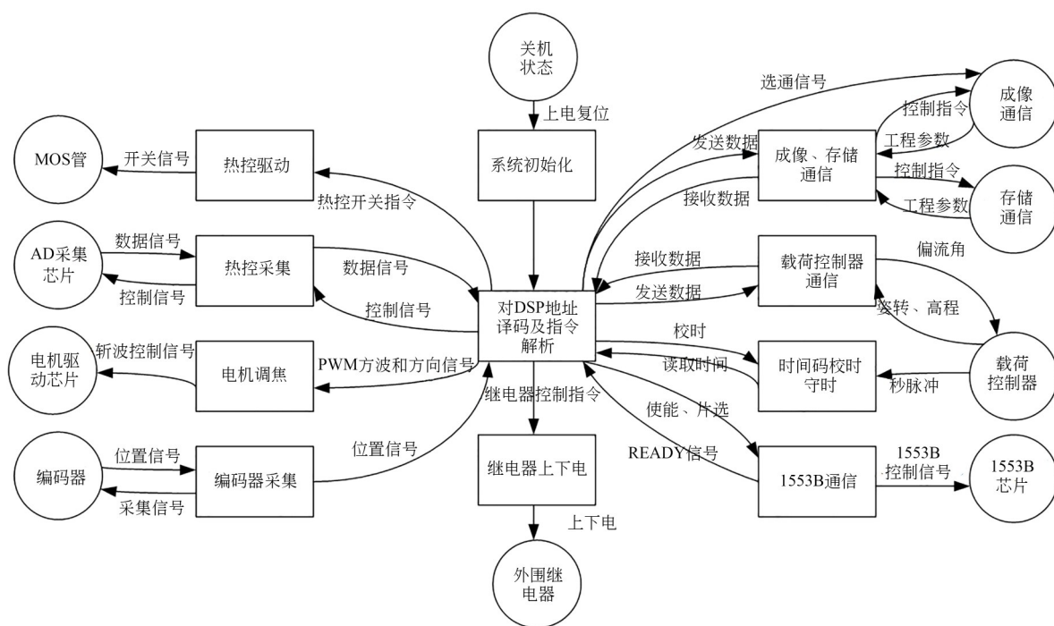
图2 主控接口扩展逻辑FPGA运行环境
