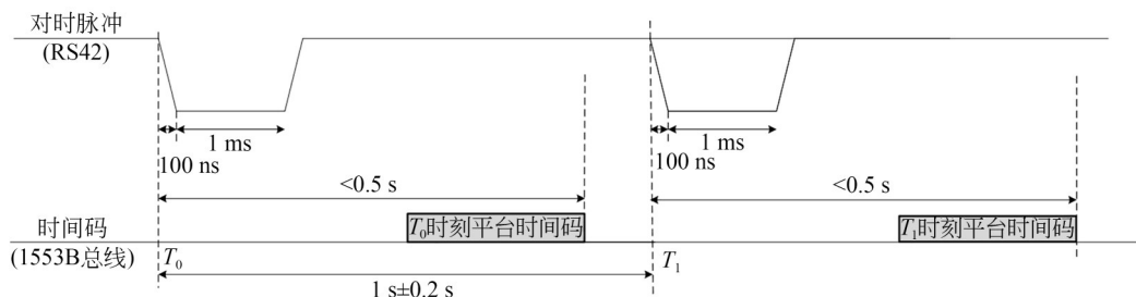
图 7 秒脉冲接口时序图
