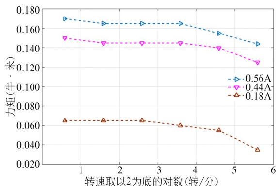
图 10 电机矩频特性曲线
